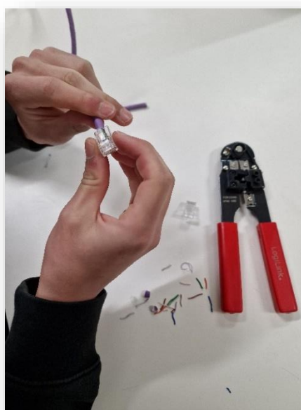
Figura 2 – Colocar a ficha RJ45
