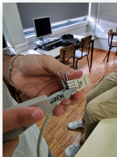
Figura 4 – Colocar os fios na ficha RJ45 fêmea
